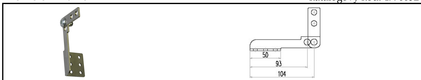
Konzole PAN K 52
