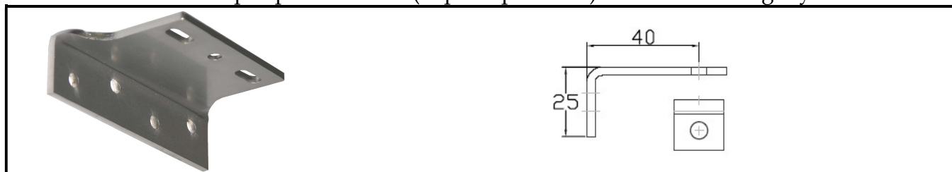
Konzole PAN K 48 - pro protikus F 14 (např. Sapa Alure)
