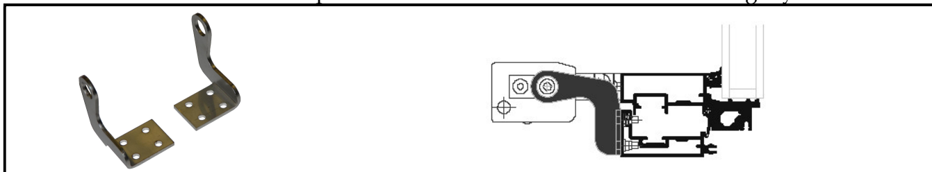
Konzole PAN K 102 - KSA na profilu Schüco AWS 102
