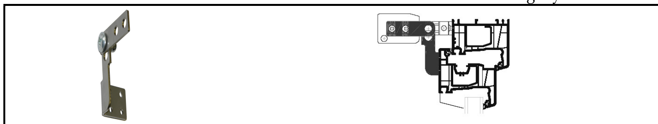
Konzole PAN K 64
