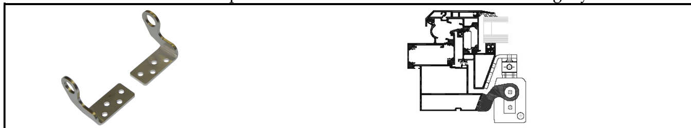
Konzole PAN K 66 - KSA na profilu Schüco AWS 57 RO
